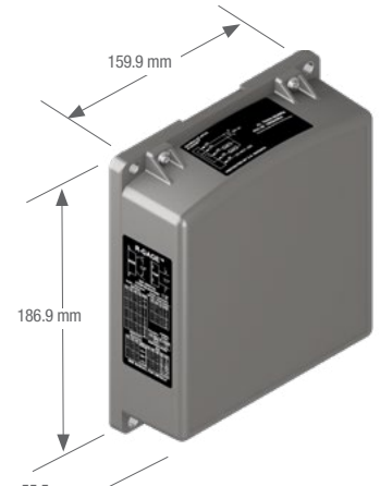
R-GAGE® Q240RA
